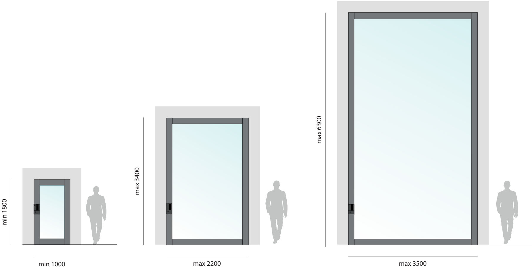
Dimensions minimales avec verre thermique pare-balles et anti masse.
